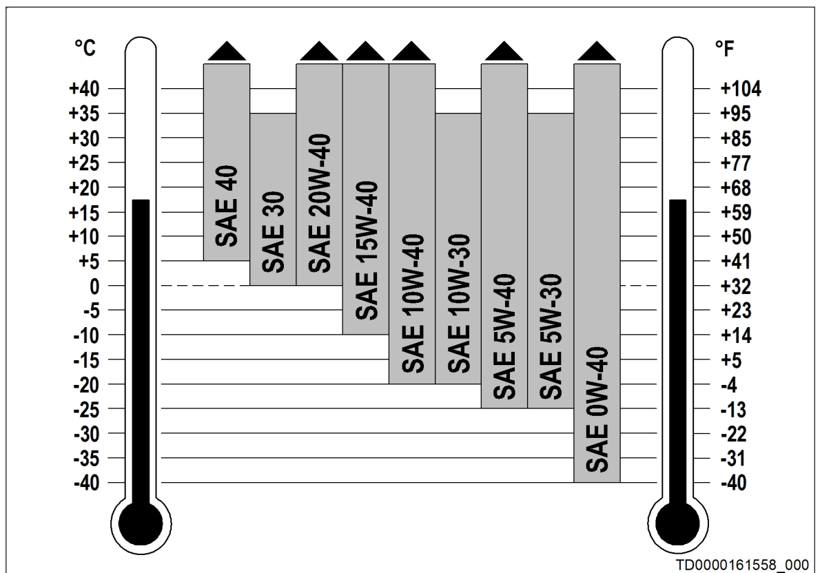
Abbildung 1: Zusammenhang der Viskositätsklassen und der Einsatztemperaturbereiche
